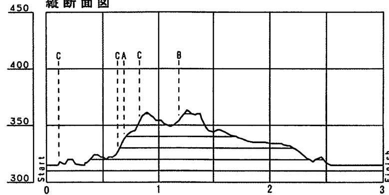
縦断面図
