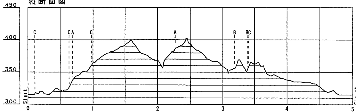
縦断面図
